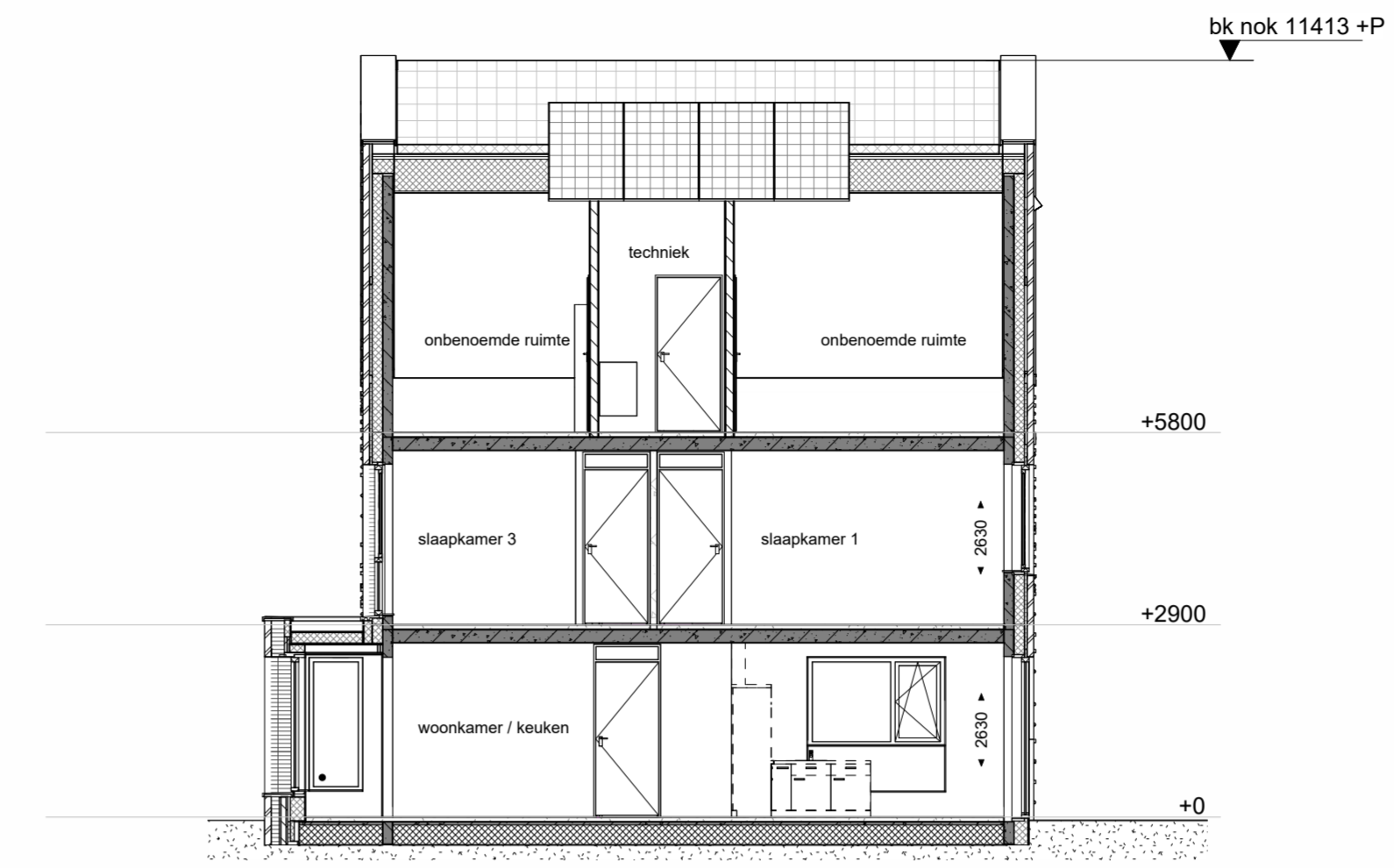
doorsnede A-A 1 : 100
