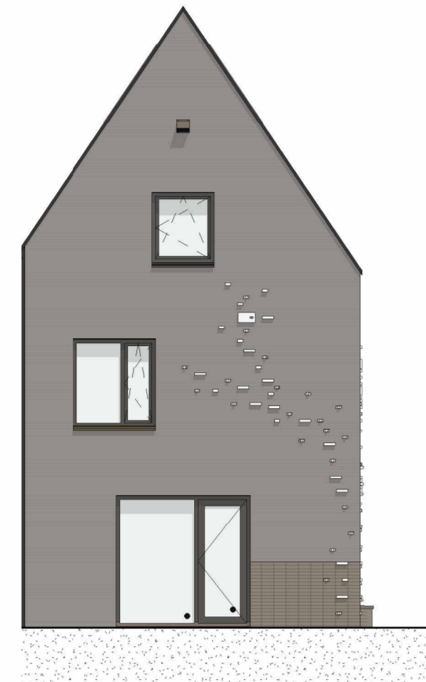
achtergevel 1 : 100
