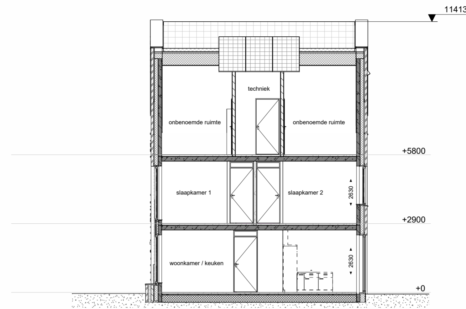
doorsnede A-A
