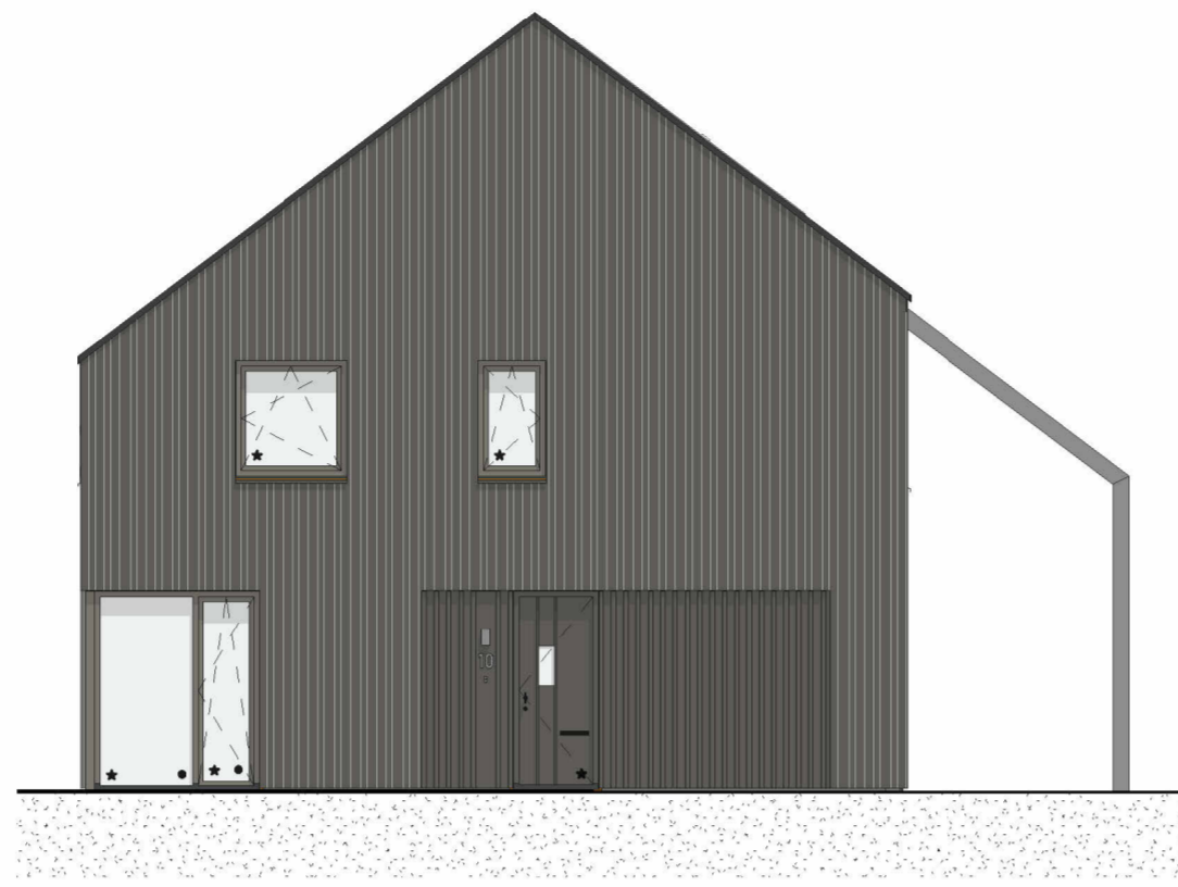
rechterzijgevel 1 : 100
