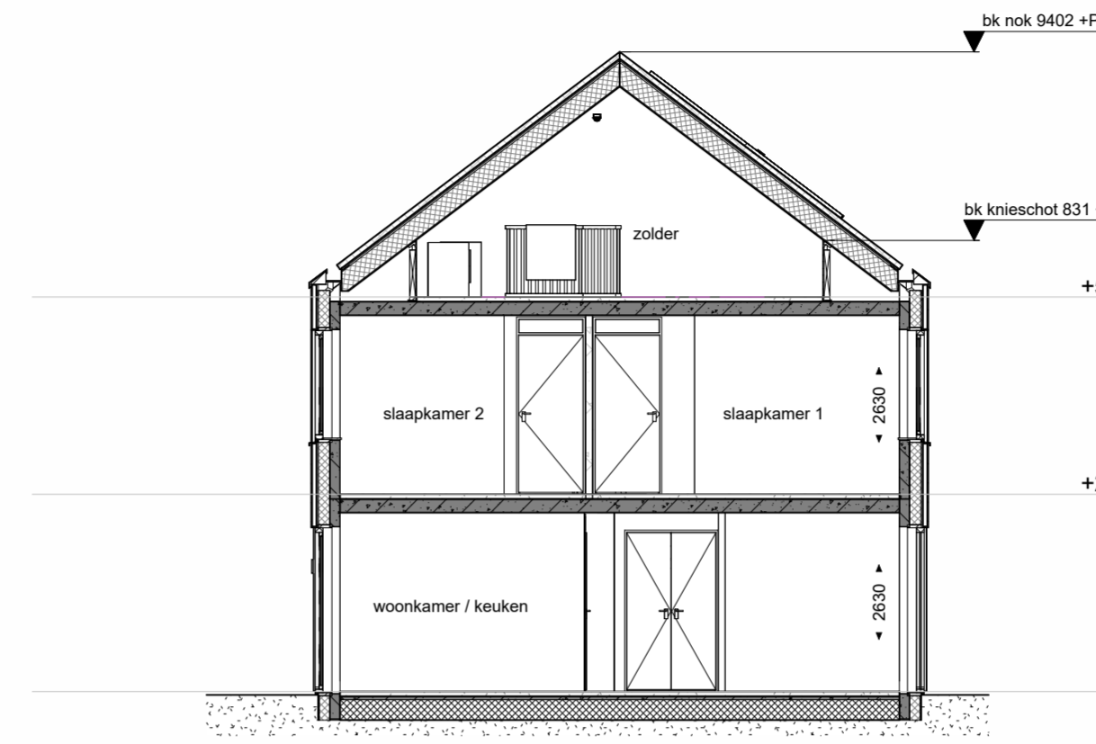
doorsnede A-A 1 : 100
